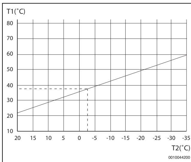
Bild 17 Radiator
