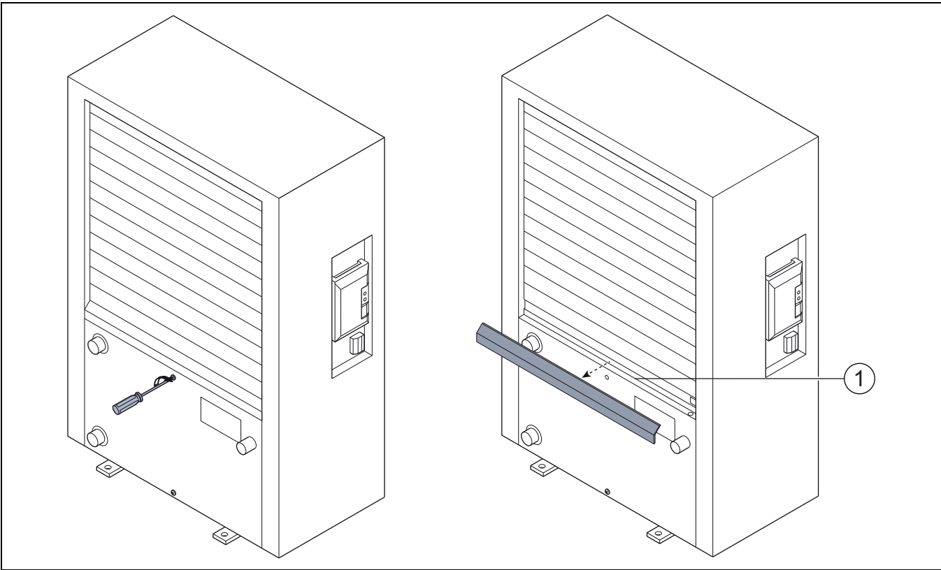
Bild 9 Värmepumpens kondenstråg
